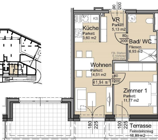
GRUNDRISS BK 01
