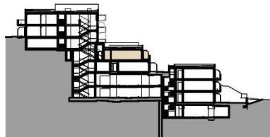
SCHNITT BK 02+04
