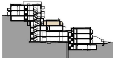
SNITT BK 02+04
