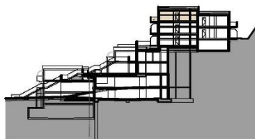
SCHNITT BK 02+04
