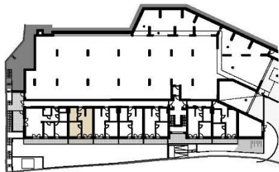
GRUNDRISS BK 01
