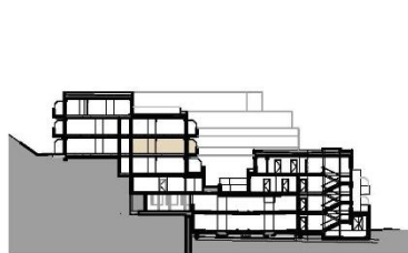
SCHNITT BK 01+03
