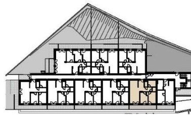
GRUNDRISS BK 03
