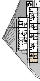
GRUNDRISS BK 03
