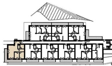
GRUNDRISS BK 03
