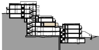
SCHNITT BK 02+04
