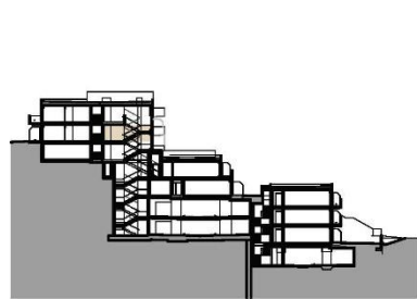
SCHNITT BK 02+04
