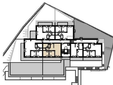
GRUNDRISS BK 04
