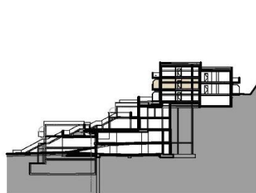
SCHNITT BK 02+04
