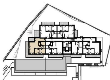
GRUNDRISS BK 04
