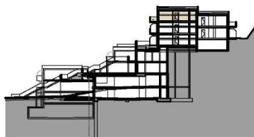
SCHNITT BK 02+04
